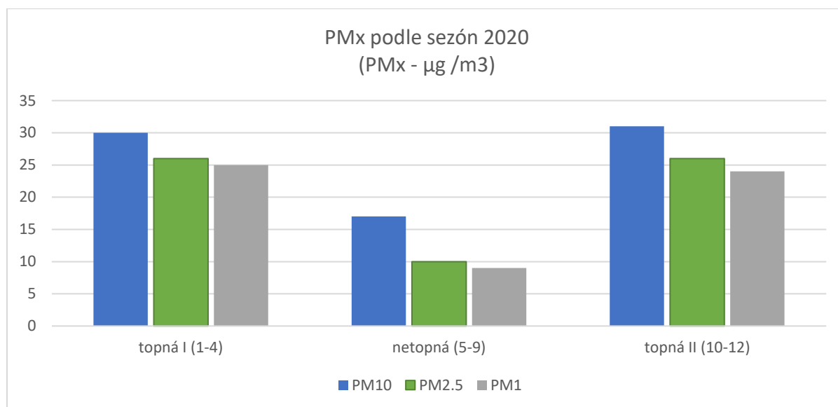
Obr. 2: Porovnání průměrných hodnot PM x podle sezón na stanici 2299.
