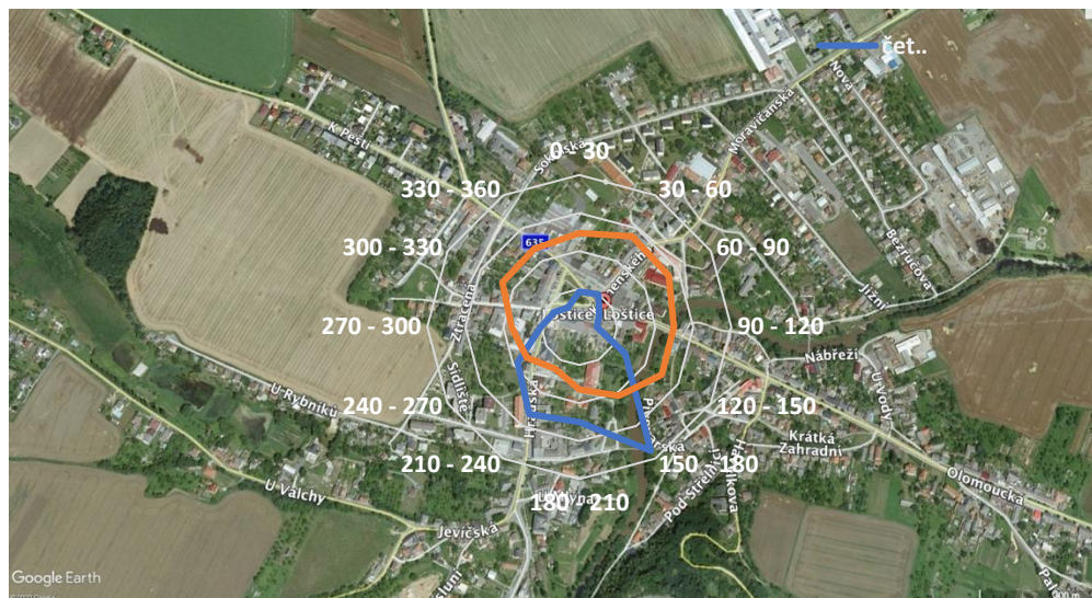
Obr. 9: Větrná růžice pro PM_{10} v Lošticích
