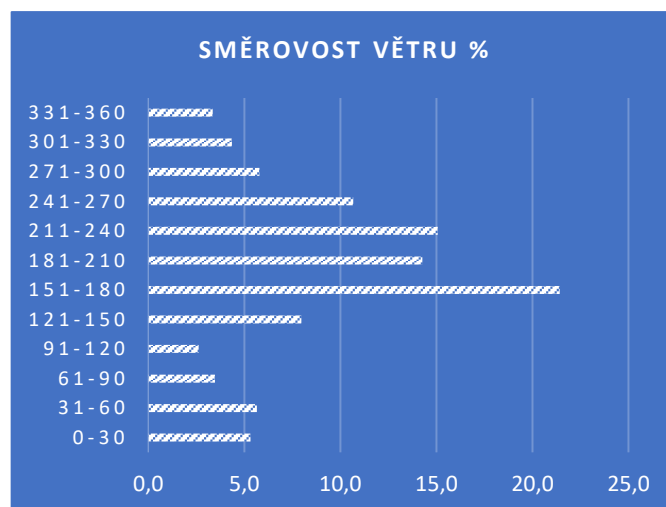
Obr. 8: Směrovost větru na stanici 2299 ve třídách po 30°.
