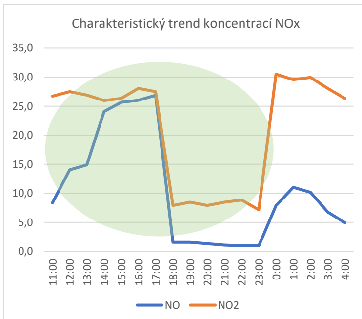
Obr. 6: Vývoj koncentrací \text{NO}_x na stanici 2299, charakteristický průběh
