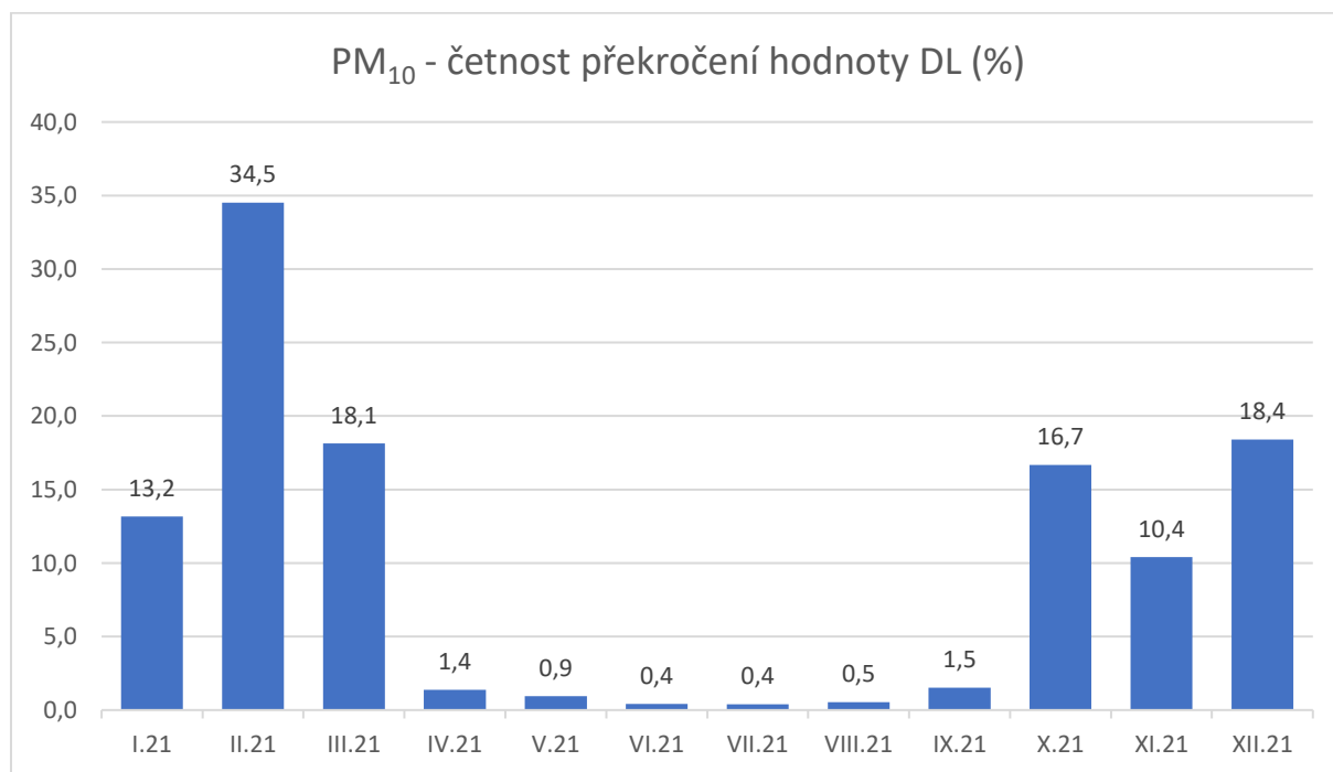
Obr.1: Četnost překročení DL v jednotlivých měsících na stanici 2299
