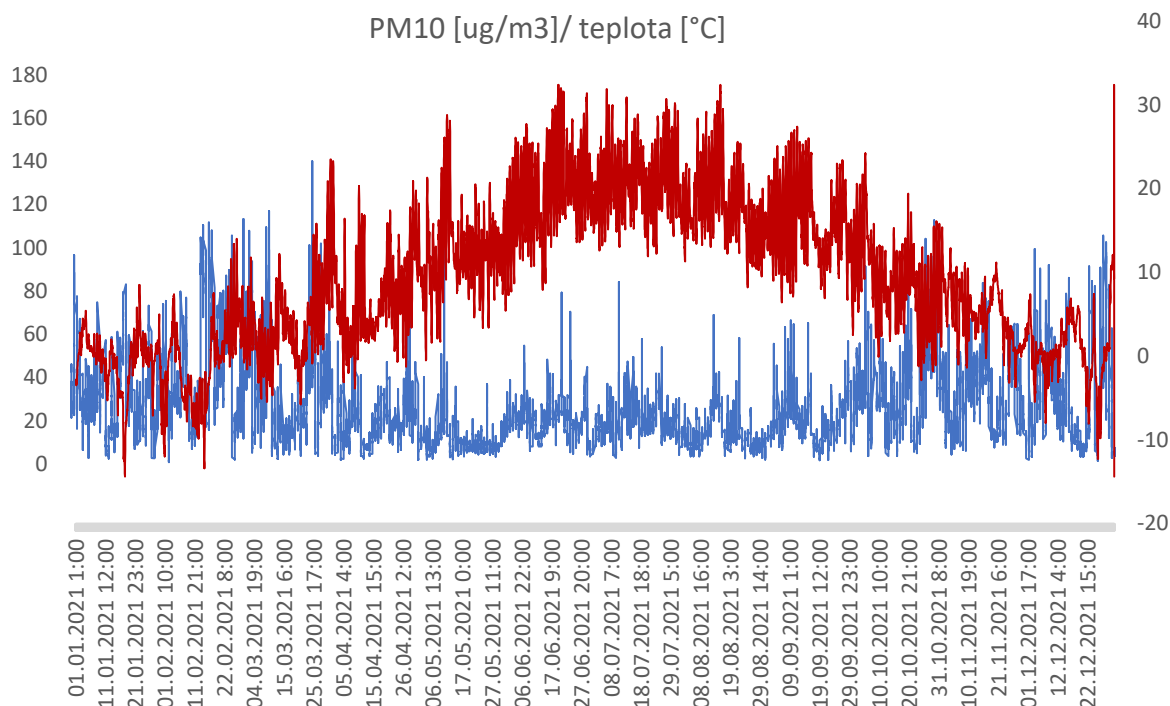
Obr. 3: Porovnání denních koncentrací PM 10 a teplot podle sezón na stanici 2299.
