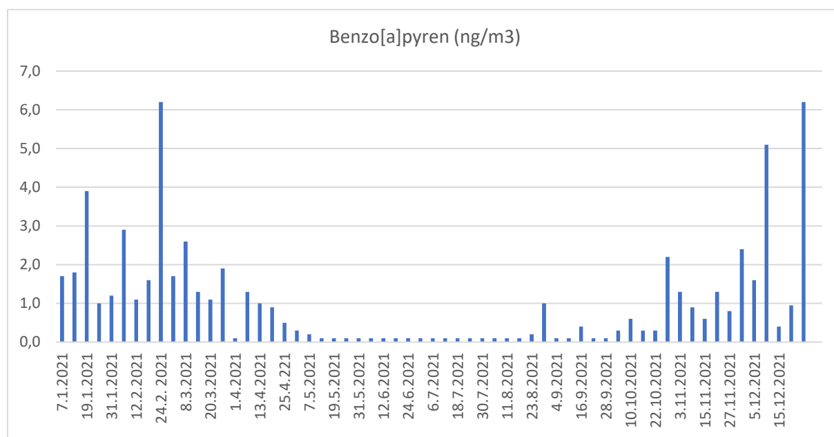
Obr. 6: Vývoj denních koncentrací benzo(a)pyrenu na stanici 2299.
