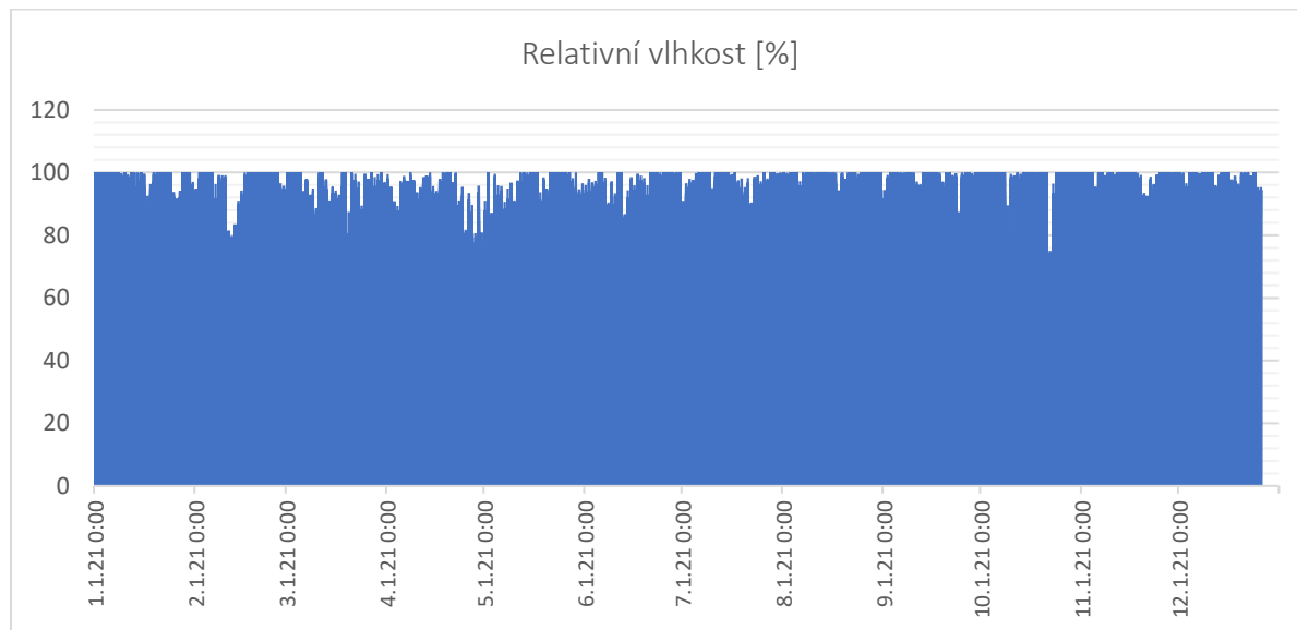
Obr. 11: Vývoj relativní vlhkosti na stanici 2299, včetně trendu.
