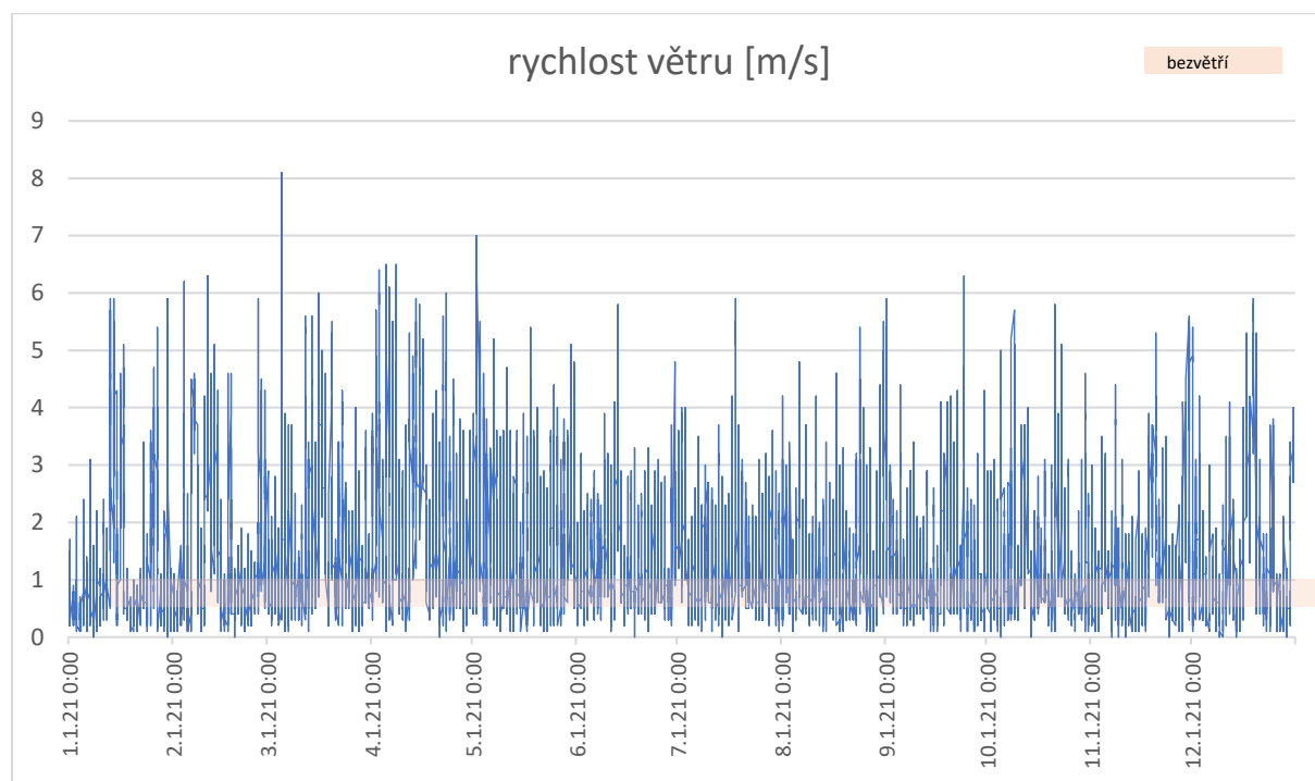
Obr. 7: Rychlost větru na stanici 2299 v hodinových údajích
