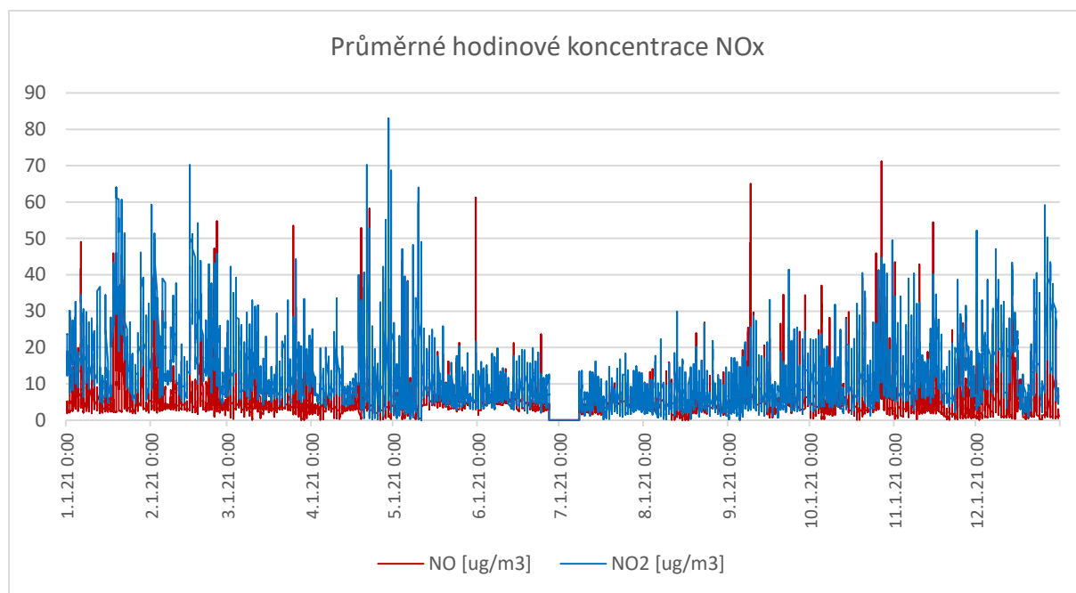
Obr. 4: Vývoj denních koncentrací NO x na stanici 2299, včetně trendu
