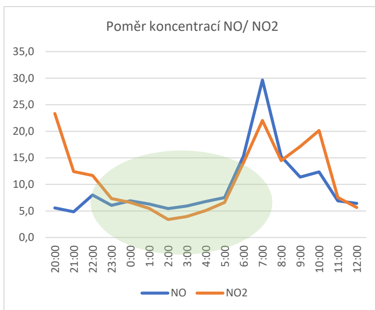
Obr. 5: Vývoj koncentrací \text{NO}_x na stanici 2299, epizoda s primárním NO
